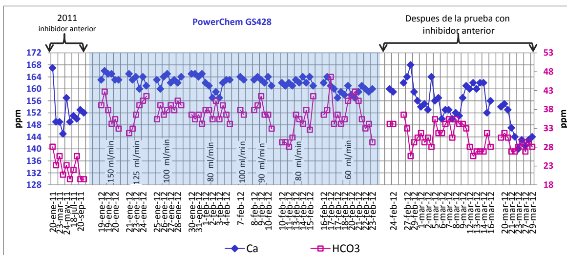
Gráfica 6. Concentración de calcio y bicarbonatos antes y después de la prueba con GS428.
