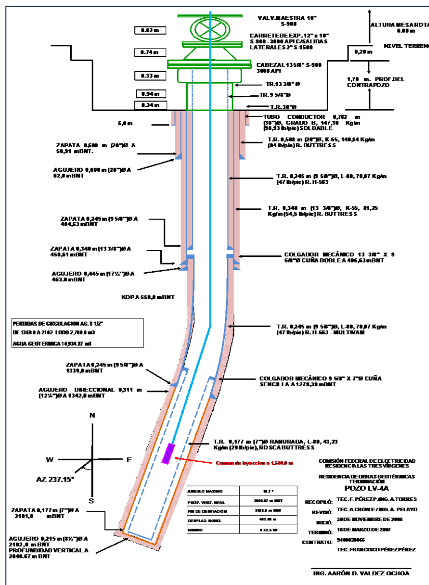
Fig. 1. Esquema del pozo LV4A y ubicación de la cámara de inhibición.
