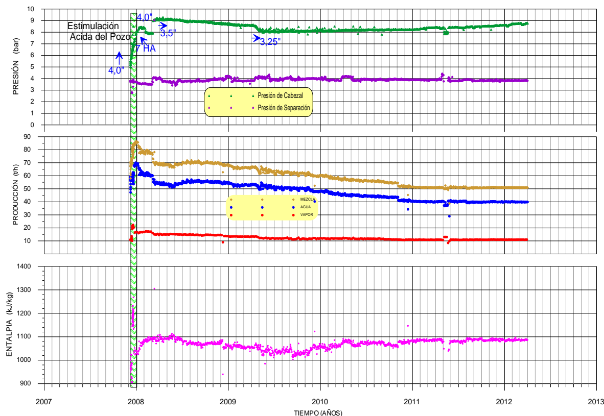
Gráfica 1. Evolución de las características de producción del pozo LV-4A
