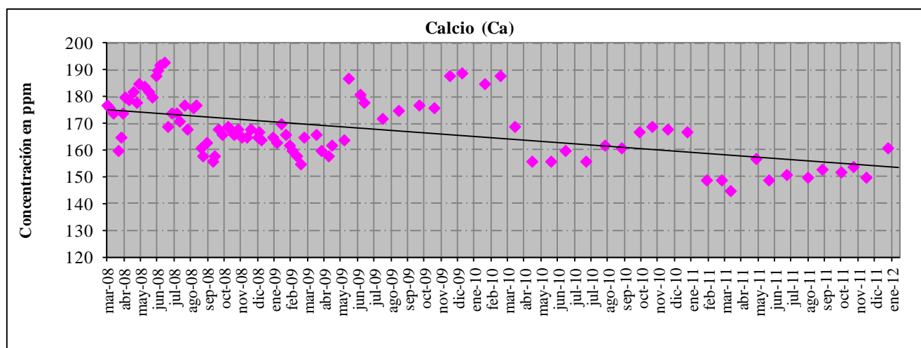
Gráfica 2. Evolución de la concentración de calcio del pozo LV-4A.
