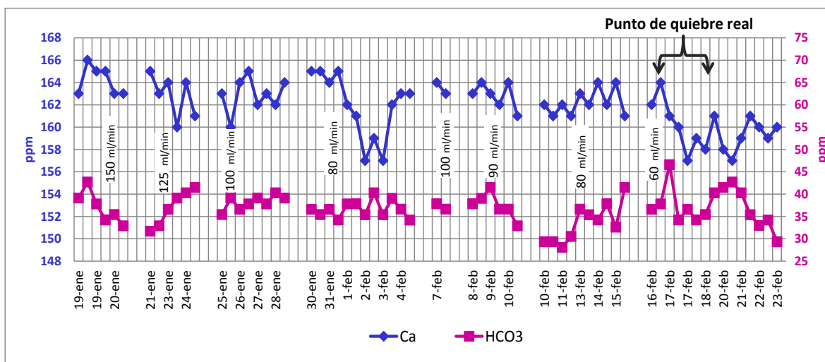
Gráfica 4. Concentración de calcio durante la segunda etapa de la prueba.
