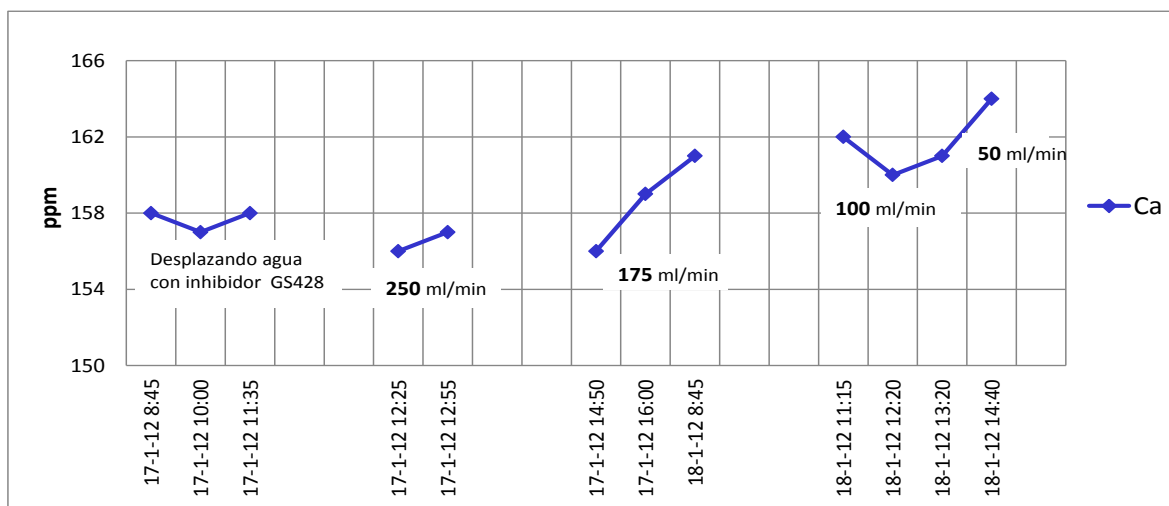
Gráfica 3. Concentración de calcio durante la primera etapa de la prueba.
