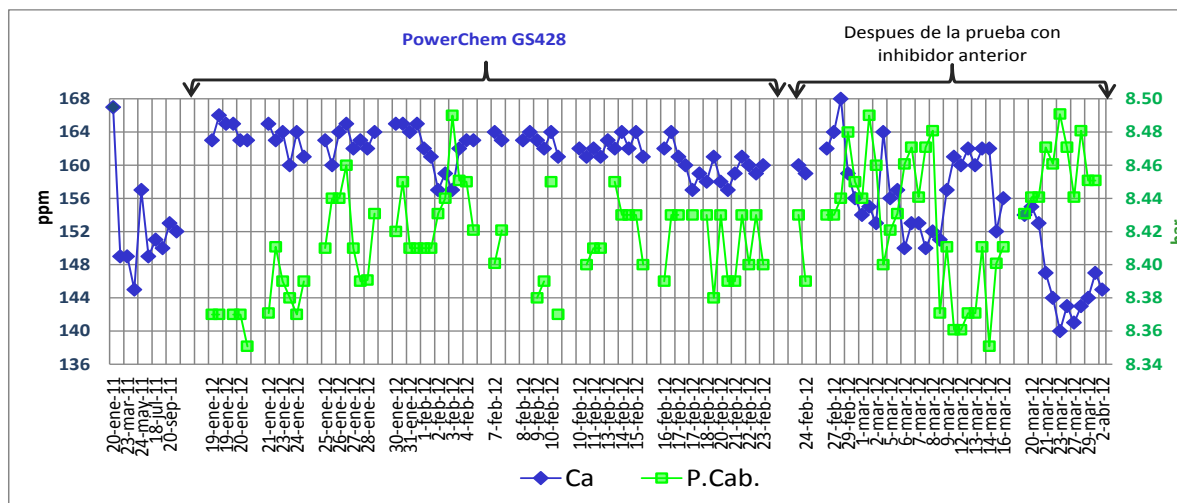
Gráfica 5. Concentración de calcio Vs Presión de cabezal.
