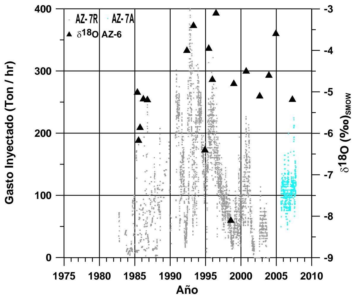
Fig. 3. Composición isotópica de \delta^{18}\text{O} del pozo AZ-6 y patrón de gastos reinyectados en el pozo AZ-7R (hasta 2003) y en el pozo AZ-7A (después de 2005).
