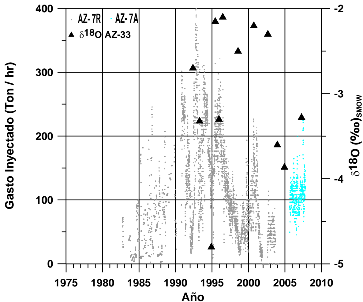
Fig. 5. Composición isotópica de \delta^{18}\text{O} del pozo AZ-33 y patrón de gastos reinyectados en el pozo AZ-7R (hasta 2003) y en el pozo AZ-7A (después de 2005).
