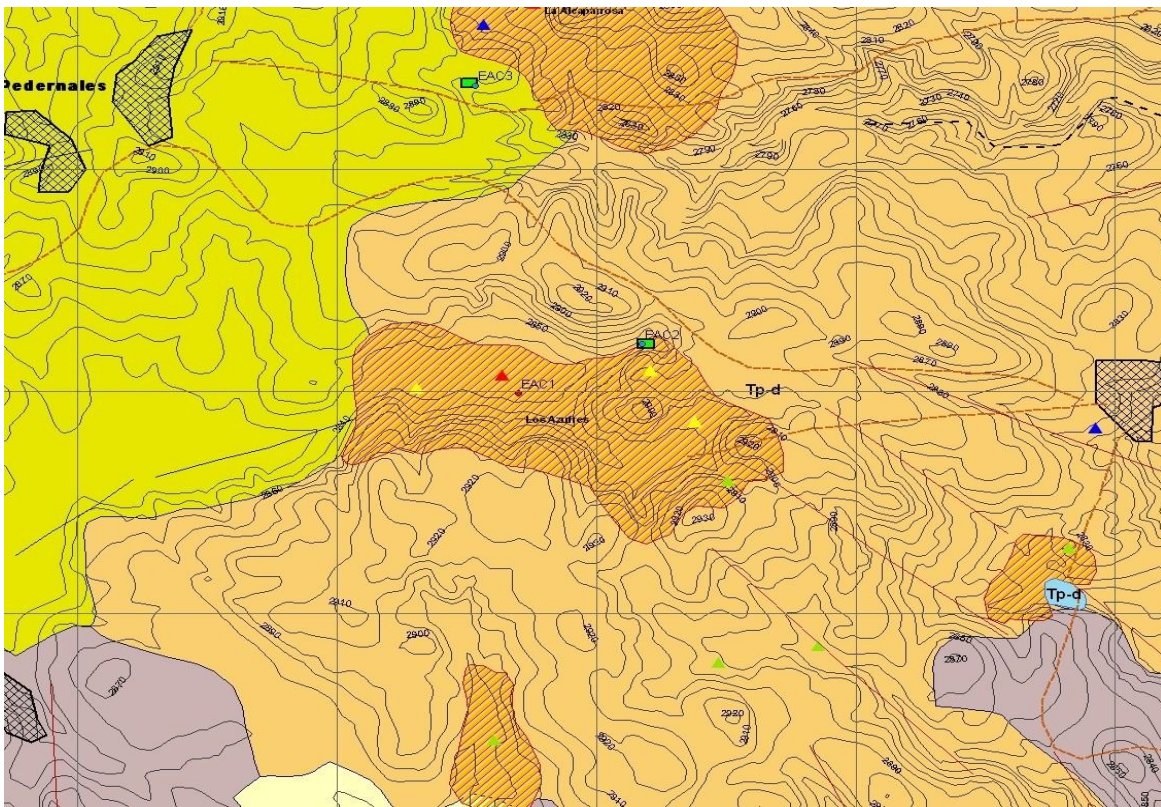
Fig. 1. Ubicación de los pozos EAC-1 y EAC-2 del área de Acapulco, Pue. (Mapa proporcionado por el ingeniero Germán Raúl Ramírez Silva).
