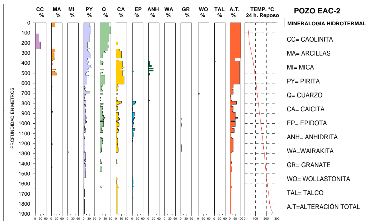
Fig. 4. Distribución porcentual y gradual de la mineralogía hidrotermal, analizada microscópicamente, y de las temperaturas (24 horas de reposo) contra la profundidad en el pozo EAC-2.
