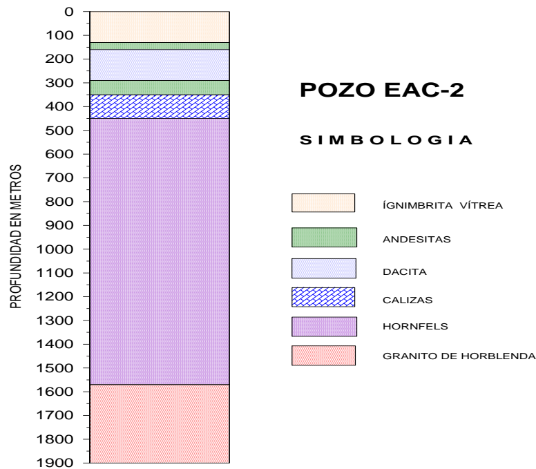
Fig. 3. Columna litológica basada en estudios microscópicos del pozo EAC-2
