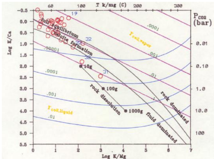
Fig. 2. Log K/Ca versus el Log K/Mg para muestras de fluidos de la región de Acoculco, Pue. (Tello-Hinojosa, 1994).
