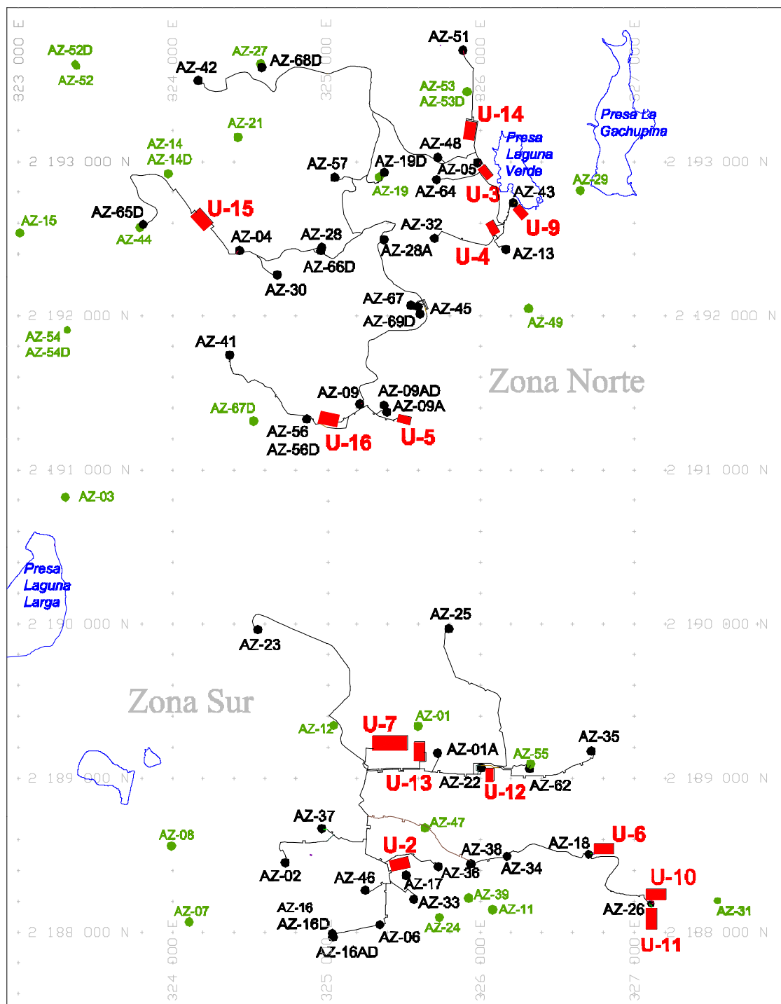
Figura 1. Red de vaporductos del campo geotérmico Los Azufres
