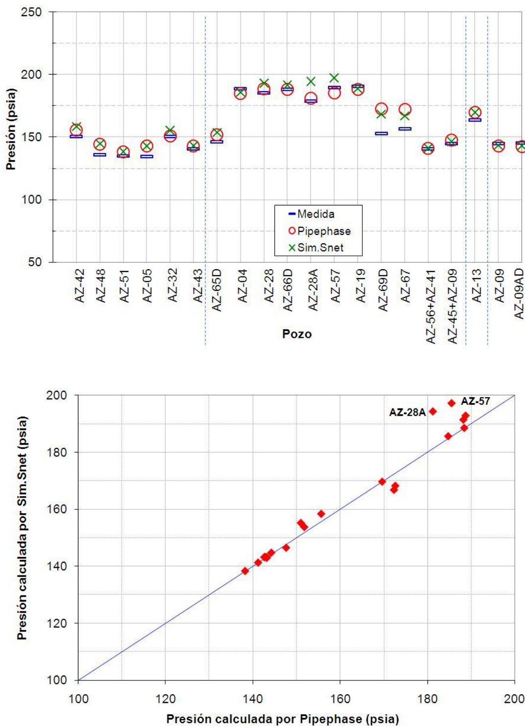
Figura 8. Presiones medidas y presiones calculadas con los simuladores Pipephase y SimSnet para los pozos de la Zona Norte. Las líneas discontinuas verticales en color azul delimitan las cuatro subredes independientes.
