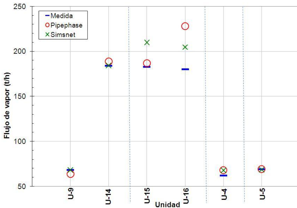
Figura 10. Comparación de flujos medidos y flujos calculados con Pipephase y SimSnet en las plantas de la Zona Norte. Los guiones verticales azules delimitan las subredes independientes.
