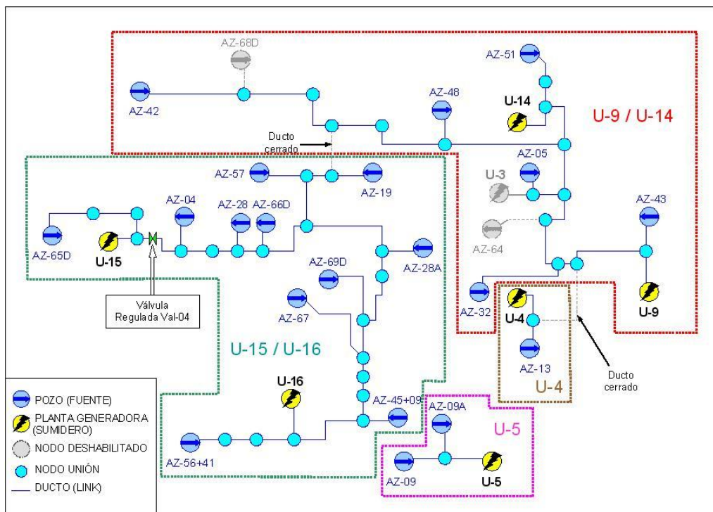
Figura 4. Diagrama del modelo de red de vaporductos de la Zona Norte del CGLA.
