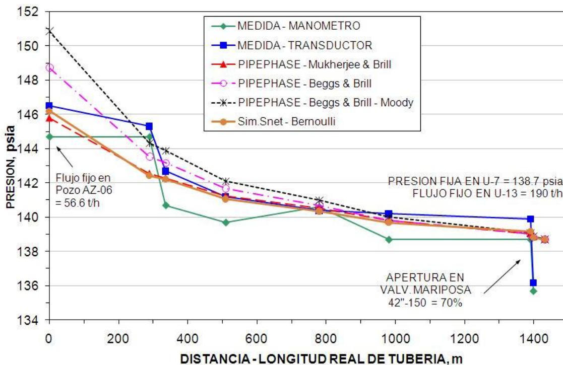
Figura 3. Ajuste de datos de presión medidos en el Colector Principal de la Zona Sur con tres métodos de cálculo de caída de presión incluidos en el simulador Pipephase.
