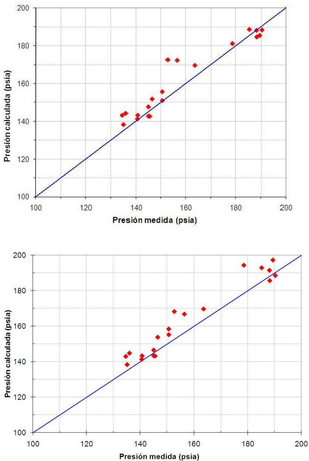
Figura 6. Comparación de presiones medidas y calculadas en pozos de la Zona Norte del CGLA, con Pipephase (arriba) y con Sim.Snet (abajo).
