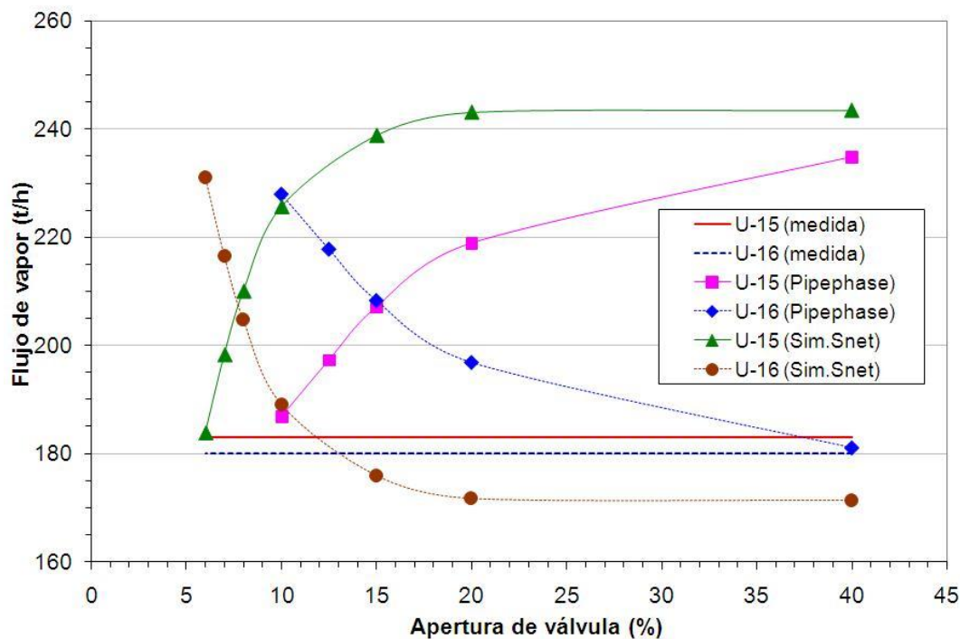
Figura 9. Variación de la producción de vapor en las unidades U-15 y U-16 en función de la apertura de la válvula Val-4.
