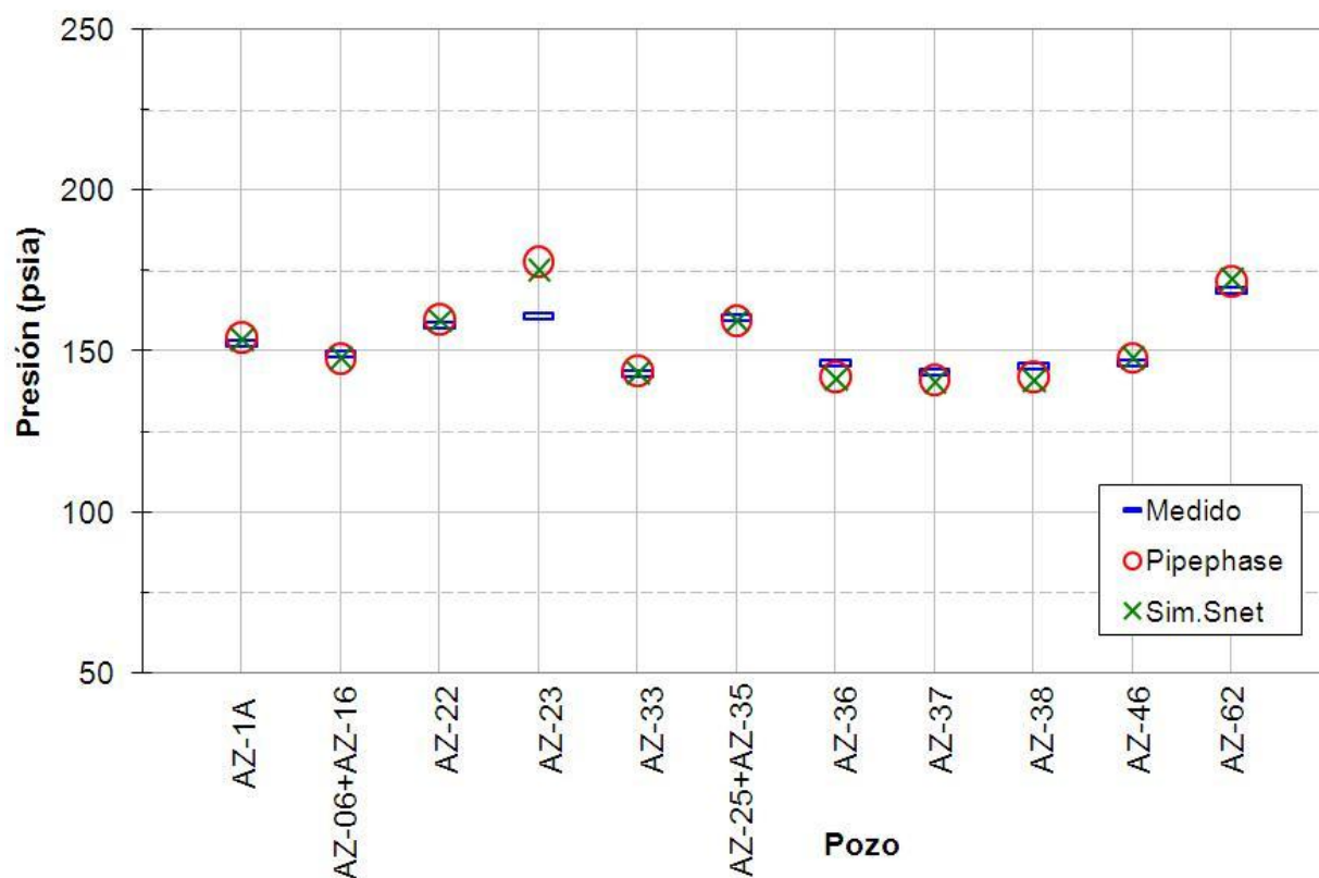
Figura 11. Comparación de presiones medidas y calculadas por Pipephase y SimSnet para los pozos de la Zona Sur.
