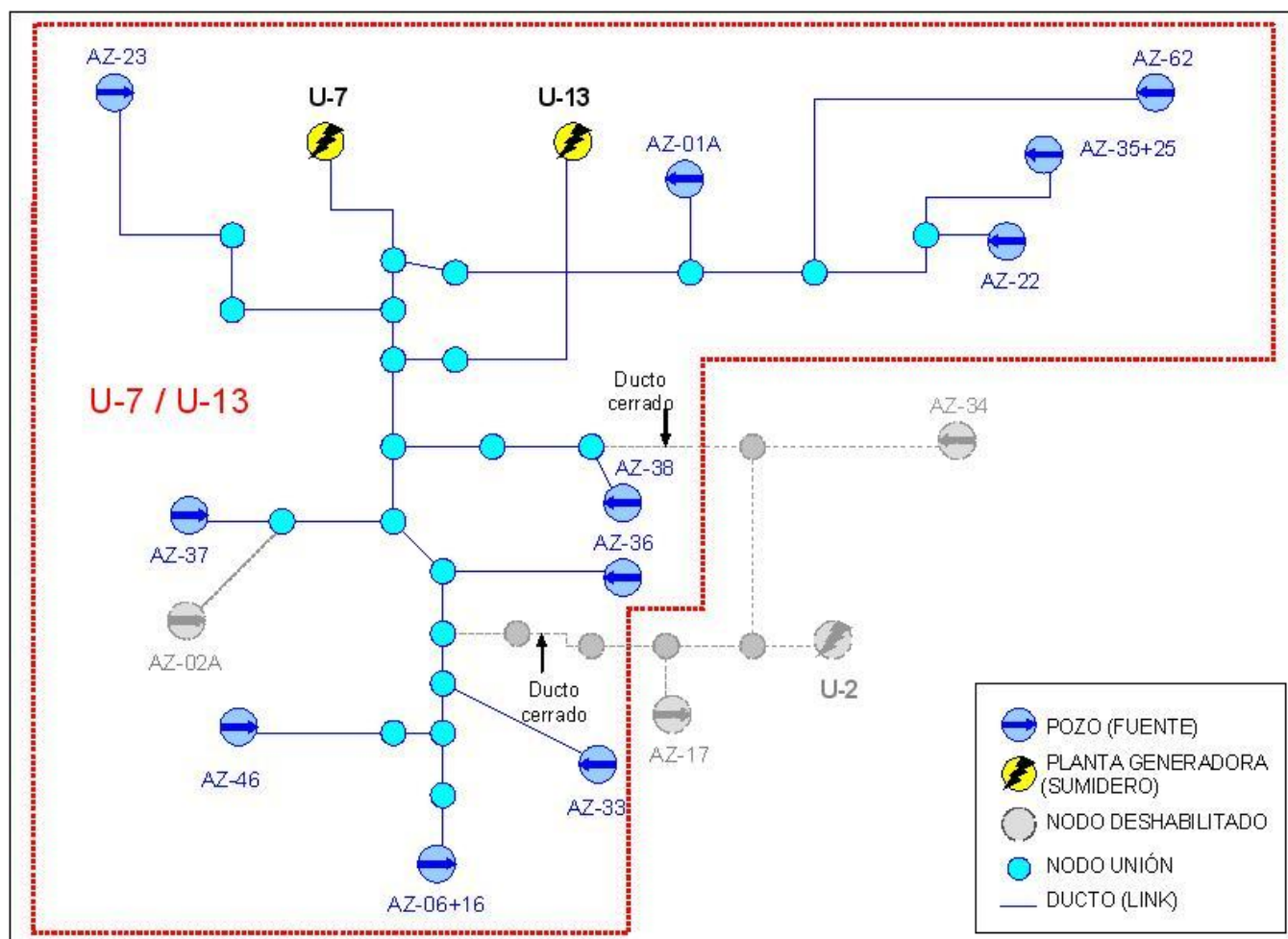
Figura 5. Diagrama del modelo de red de vaporductos de la Zona Sur del CGLA
