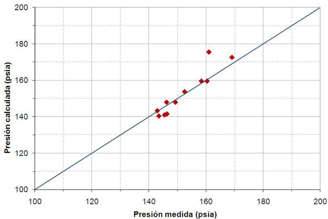
Figura 7. Comparación de presiones medidas y calculadas en pozos de la Zona Sur del CGLA, con Pipephase (arriba) y con Sim.Snet (abajo).
