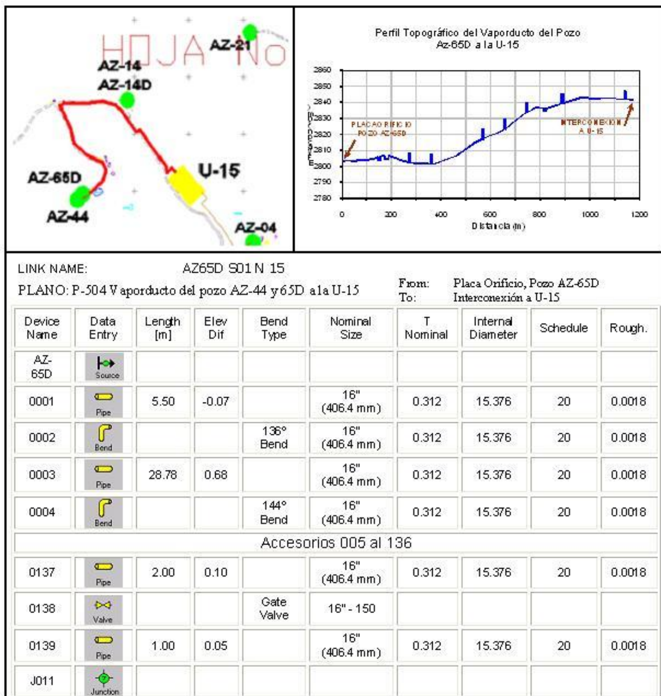
Figura 2. Ejemplo de formato de documentación del modelo de la red de vapor ductos del CGLA
