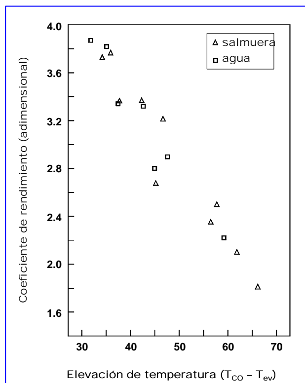
Fig. 6. Variación del coeficiente real de rendimiento como función de la elevación total de temperatura de la BC por compresión mecánica (Frías et al., 1991)
