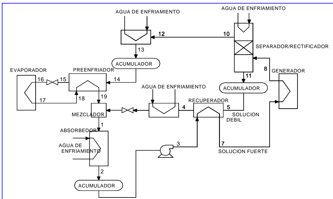
Fig. 2. Esquema de la BC por absorción amoníaco/agua probada para refrigeración en los campos geotérmicos de Los Azufres y Cerro Prieto (Best et al., 1986; 1990)
