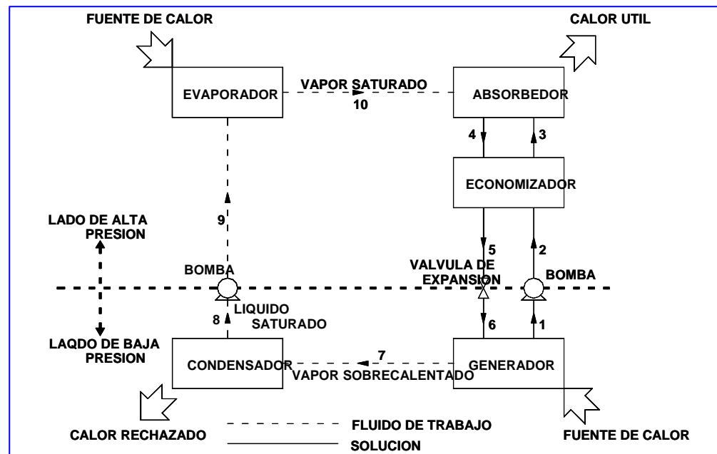
Fig. 2. Esquema de la BC por absorción amoníaco/agua probada para refrigeración en los campos geotérmicos de Los Azufres y Cerro Prieto (Best et al., 1986; 1990)
