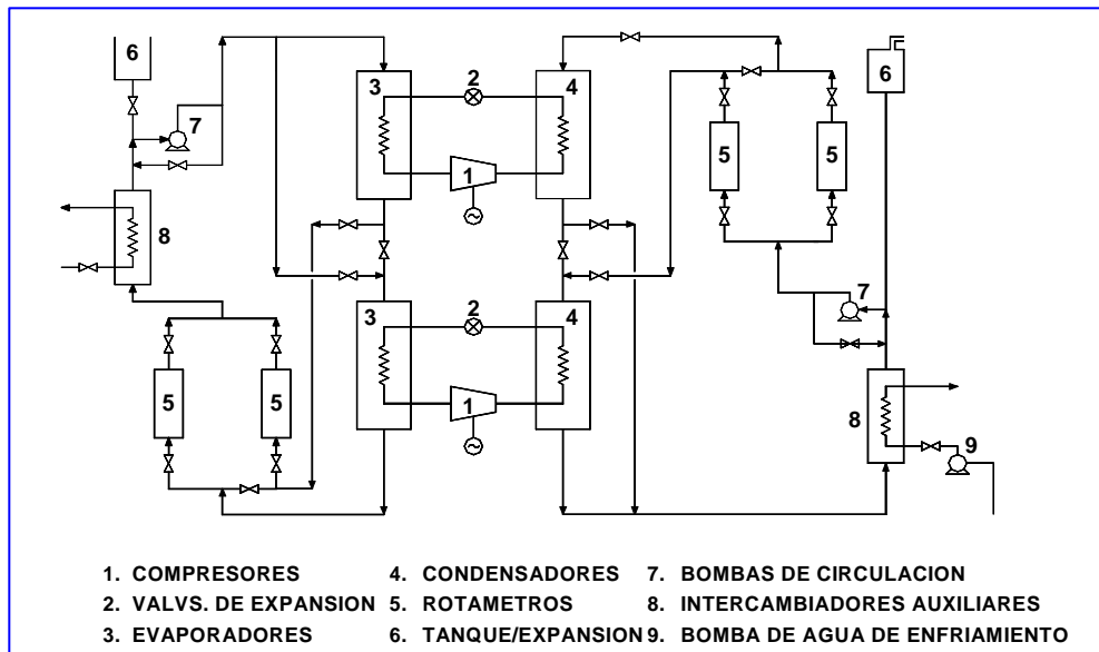
Fig. 4. Arreglo esquemático de la BC por compresión mecánica probada en el campo geotérmico Los Azufres (Frías et al., 1991)
