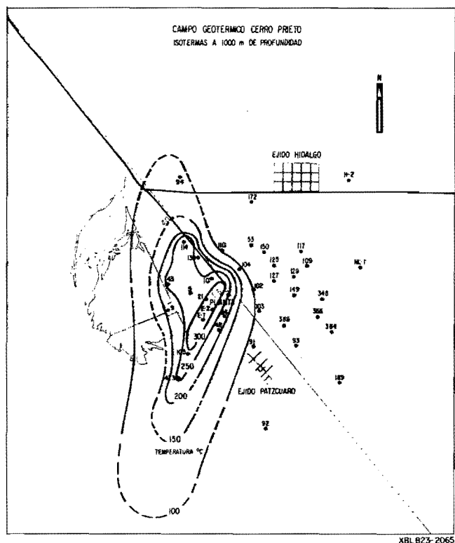
Figura 10. Mapa mostrando la configuración de las isotermas a 1000 m de profundidad.
