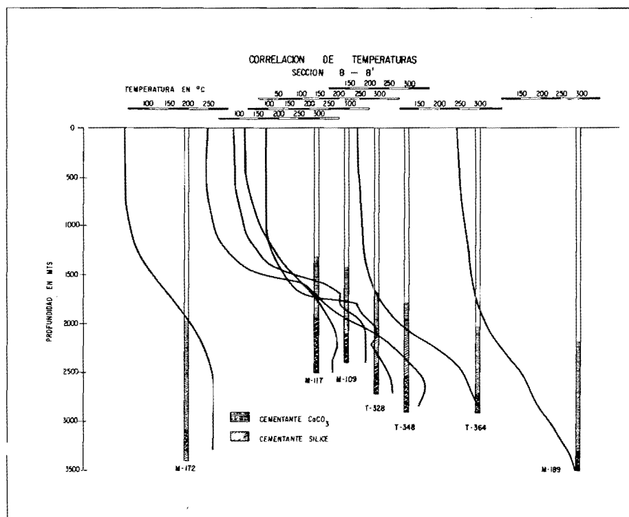
Figura 3. Correlación de temperaturas. Sección B-B'.
