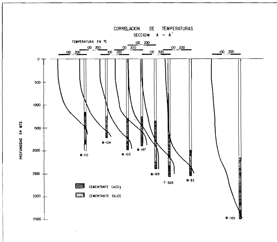
Figura 2. Correlación de temperaturas. Sección A-A'.
