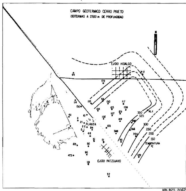
Figura 13. Mapa mostrando la configuración de las isotermas a 2500 m de profundidad.
