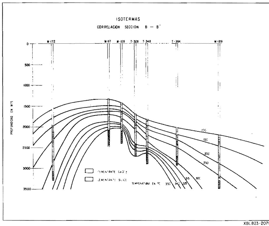
Figura 5. Isotermas. Sección B-B'.
